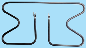
Arçelik Tost Rezistansı 110V. 800W (6.5 Ø-Cr-ni)
