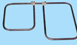
Tost Rezistansı 110V. 800W (6.5 Ø-Cr-ni)
