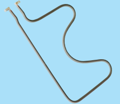
Ultra Tost Rezistansı 110V. 900W (6.5 Ø-Cr-ni)
