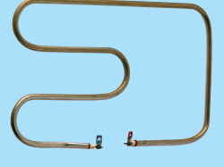
Arçelik Tost Rezistansı CR 115 137 110 V. 1000 W. (6.5 Ø-Cr-ni)
