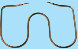
Tost Rezistansı CR 115 139 110 V. 1000 W. (6.5 Ø-Cr-ni)
