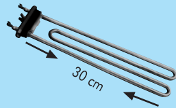
AEG/ARÇELİK Çam. Mk. Rez. 220V. 2000W (8.5 Ø-Cr-ni) CR 116 245
