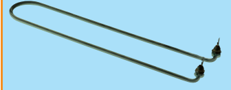
Benmari Rezistansı (Kıvrık) CR 115 821 40-50-60 cm= 220V. 1500W (8.5 Ø-Cr-ni)
