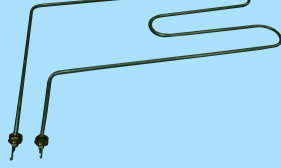
Benmari Rezistansı 220V. 2500W (8.5 Ø-Cr-ni)
