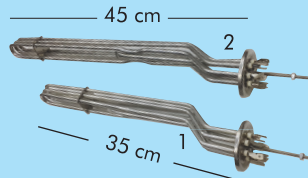
Yuvarlak Flaşlı BYM Rezistansı 380/220V. 3x3000W (6.5 Ø-Cr-ni) (Kısa (1) - Uzun (2))
