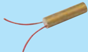
CR 113 125 Pano Fişek Rezistanslar 220V.-100W Boy:65 mm Çap:16mm
